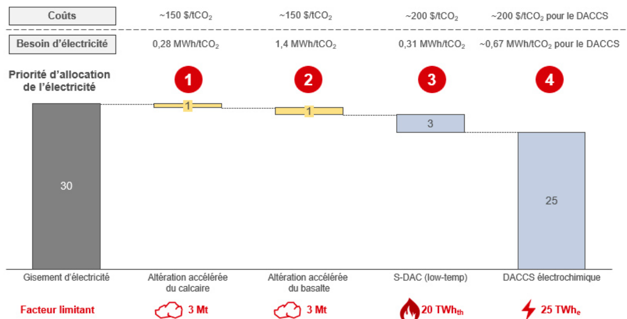
Figure 71 – Répartition du gisement d'électricité parmi les différentes méthodes d'EDC consommant de l'électricité dans le scénario ambition en 2050 [TWh/an]
