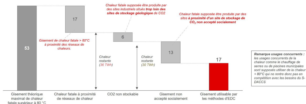
Figure 47 – Estimation du gisement de chaleur fatale disponible pour l'EDC en 2050 dans le scénario de référence, [TWh/an]
