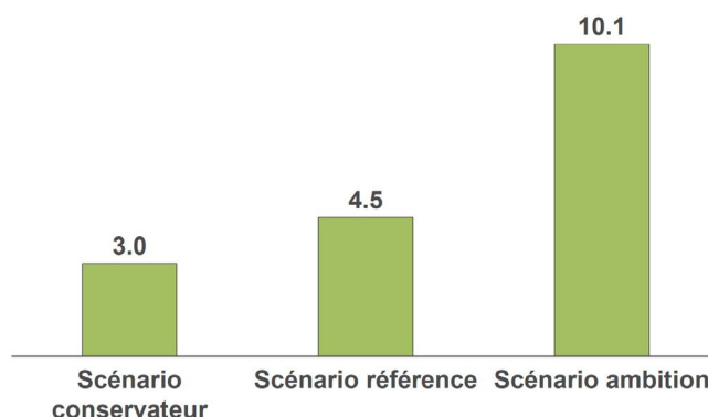
Figure 58 – Potentiel d'élimination de CO 2eq de l'afforestation selon les scénarios, en 2050 en MtCO 2eq /an
