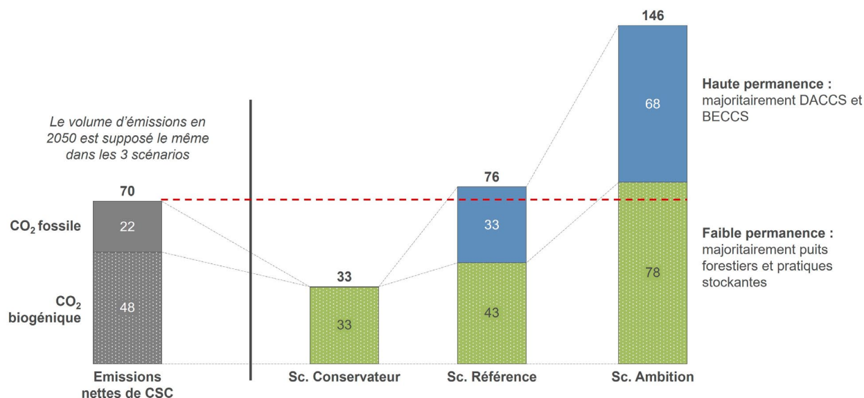
Figure 43 – Comparaison de l'origine des émissions résiduelles avec la permanence des puits de carbone mobilisés dans les trois scénarios considérés
